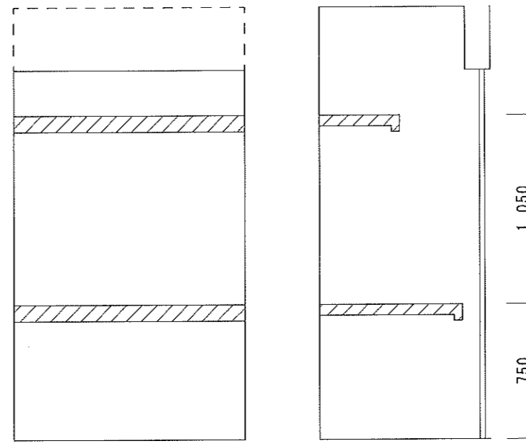
主寝室 押入2
